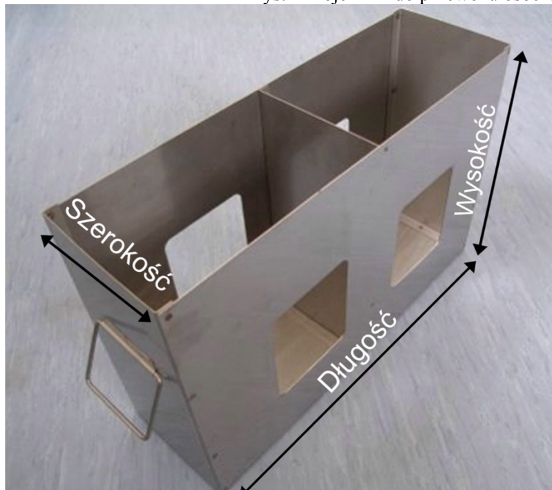
Rys. 1 Pojemnik do przewożenia osocza
